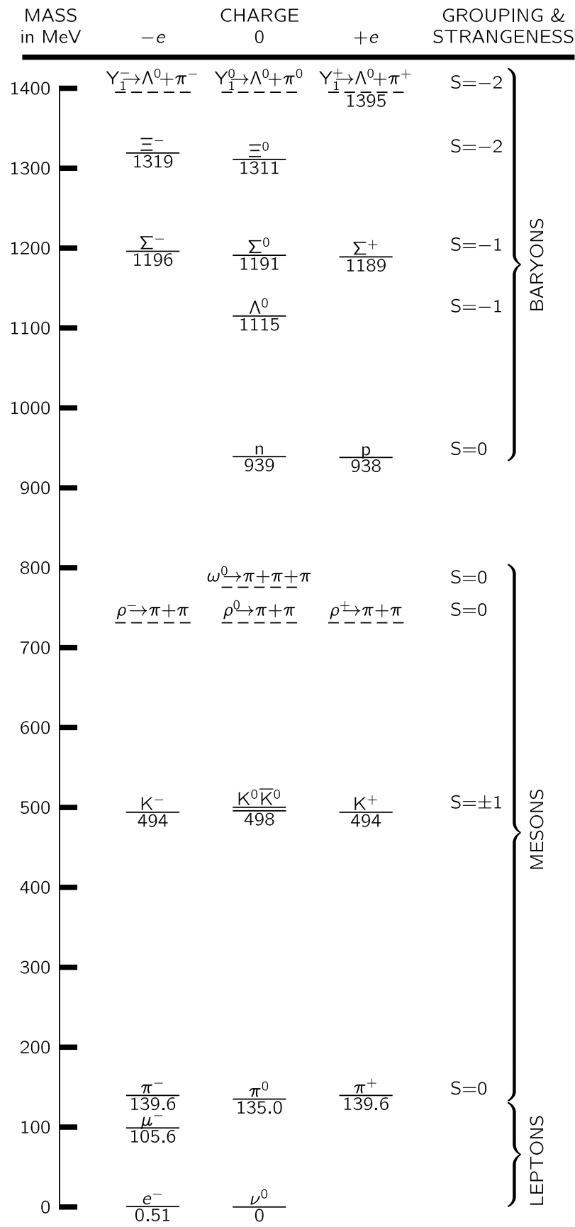
图 2.1: 基本粒子
