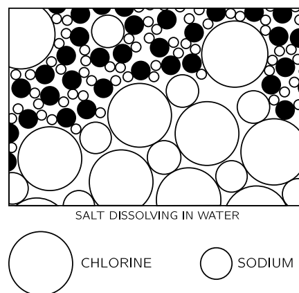
图 1.6: 盐在水中的溶解
