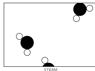
图 1.2: 水蒸气
